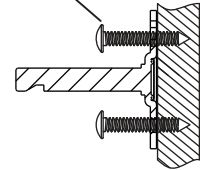
Wood Screw Tornillo para Madera Vis à bois
